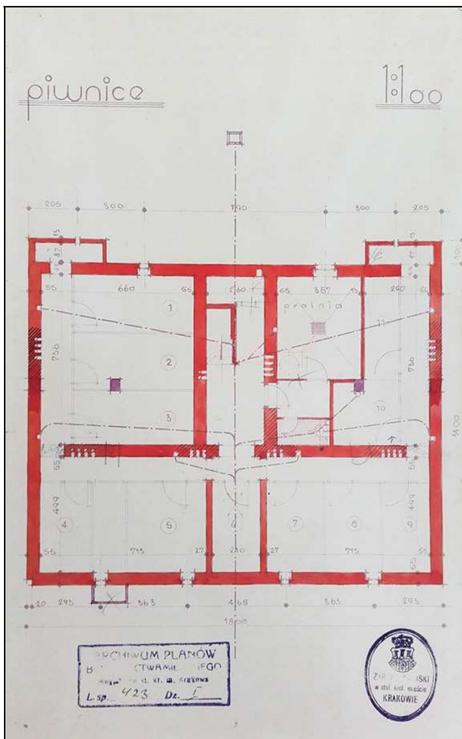
II. nr 8. Kraków, ul. św. Marka 35. Projekt istniejącej kamienicy, rzut piwnic. Bachner, M. Stiel, 1935 r. ABM, f. 573 a. | Fot. M. Goras
