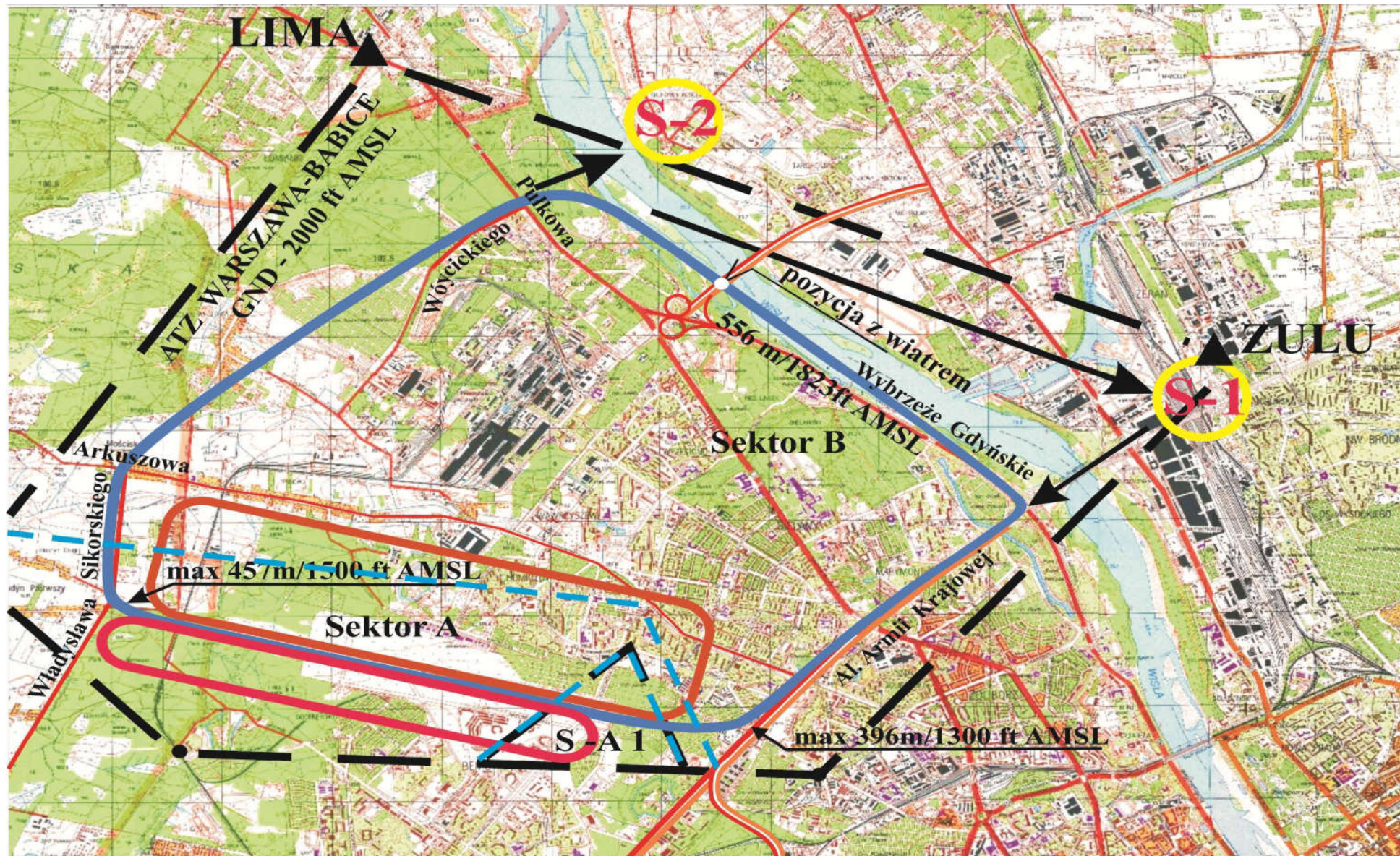
Samolotowy i szybowcowy krąg nadlotniskowy na lotnisku Warszawa-Babice.
